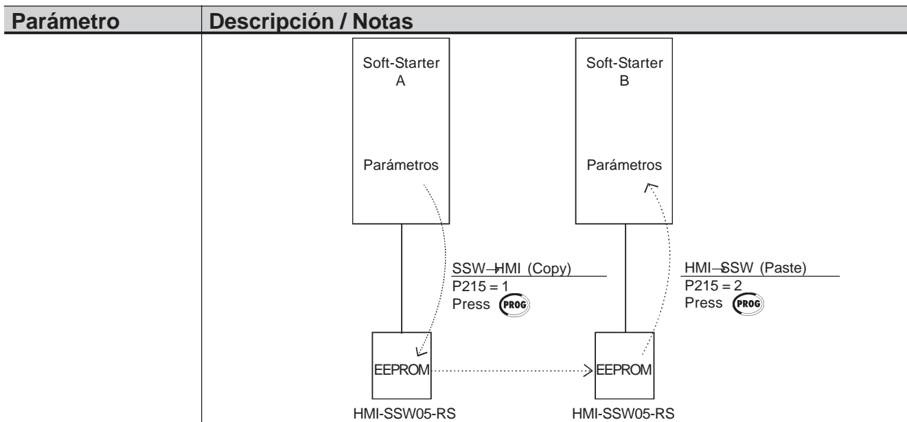
Figura 22.2 - Copia de la parametrización de la Soft-Starter A para la Soft-Starter B utilizando la función copy y HMI-SSW05-RS
