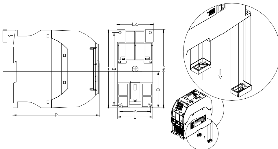
Figura 10.1 - Dimensiones de la SSW-05 Plus
